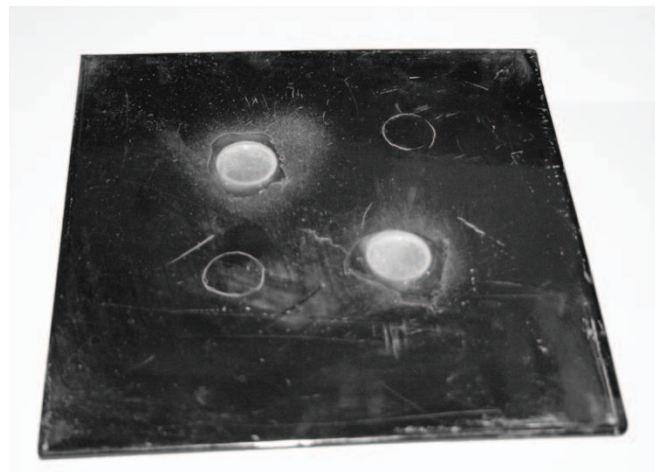
شکل ۲- نمونه‌ای از پوشش پلی یورتان ۲ پس از آزمون چسبندگی (رنگ سفید متالیک داخل حفره‌ها نشانه کنده شدن کامل پوشش از سطح می‌باشد)
