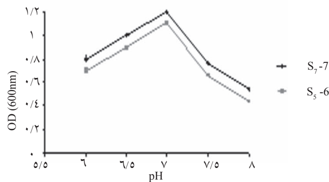
شکل ۳- بهینه‌سازی pH
