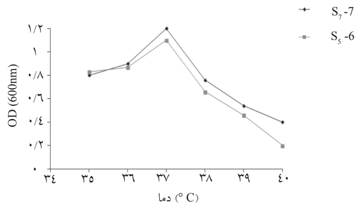
شکل ۴- بهینه‌سازی دما
