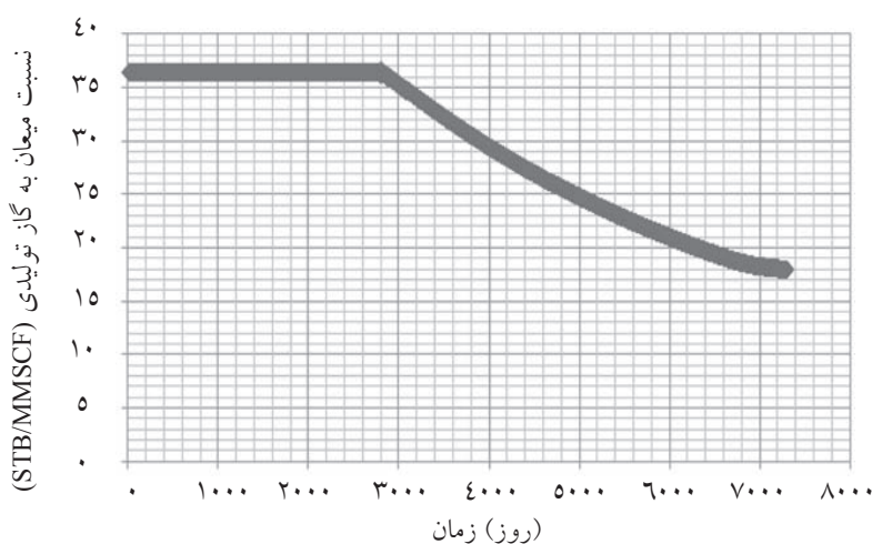
شکل ۱- تغییرات نسبت CGR با زمان در یک مخزن گاز میعانی کم مایه با شرایط ابتدایی زیر اشباع
