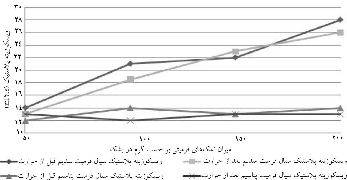
شکل ۲- تأثیر مقادیر مختلف نمک‌های فرمت سدیم و پتاسیم بر گرانروی پلاستیک سیال قبل و بعد از حرارت دادن در دمای 121^{\circ}\text{C} به مدت ۱۶ ساعت
