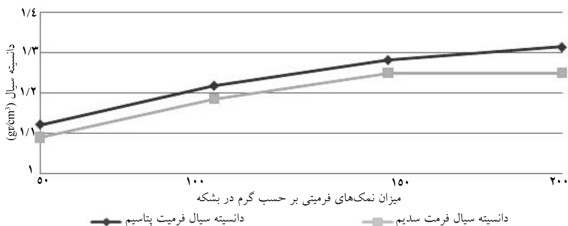
شکل ۱- تأثیر میزان نمک‌های فرمیتی سدیم و پتاسیم بر دانسیته سیال
