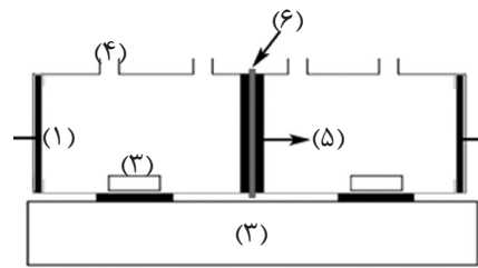
شکل ۲- شمایی از سل مورد استفاده در اندازه‌گیری خواص الکتروشیمیایی غشای تبادل یون (۱) الکتروود پلاتین، (۲) مگنت، (۳) همزن، (۴) روزنه خوراک، (۵) واشر لاستیکی و (۶) غشاء
