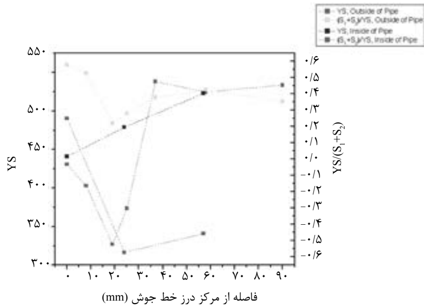
شکل ۶ تغییر مقاومت تسلیم و نسبت جمع تنش‌های پسماند سطحی بر مقاومت تسلیم در سطوح داخلی و خارجی لوله.
