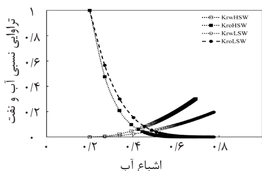
شکل ۱ نمودار تراوایی نسبی برای دو حالت HSW و LSW
