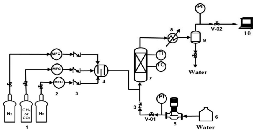
شکل ۱ نمایشی از سیستم ریفرمینگ بخار آب با متان، ۱- کپسول‌های گاز، ۲- کنترل‌کننده دبی جرمی، ۳- شیر یک طرفه، ۴- مخلوط‌کننده گازها، ۵- پمپ سوزنی، ۶- مخزن آب، ۷- کوره و راکتور، ۸- مبدل حرارتی، ۹- جداکننده فازی. PI: نشانگر فشار، TI: نشانگر دما، TC: کنترل‌کننده دما.
