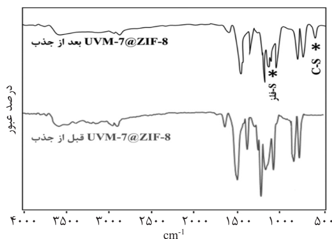
شکل ۷ طیف‌های FT-IR مربوط به UVM-7@ZIF-8 قبل و بعد از جذب DBT
