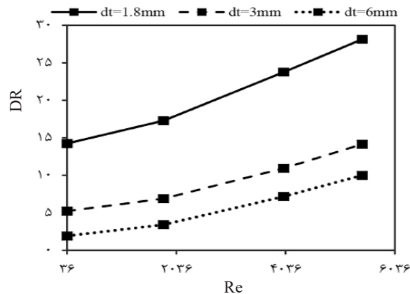
شکل ۱۰ نسبت تقسیم جریان بین دو مسیر اصلی و کنارگذر برحسب عدد رینولدز در چینش مربعی برای مقادیر مختلف d_p
