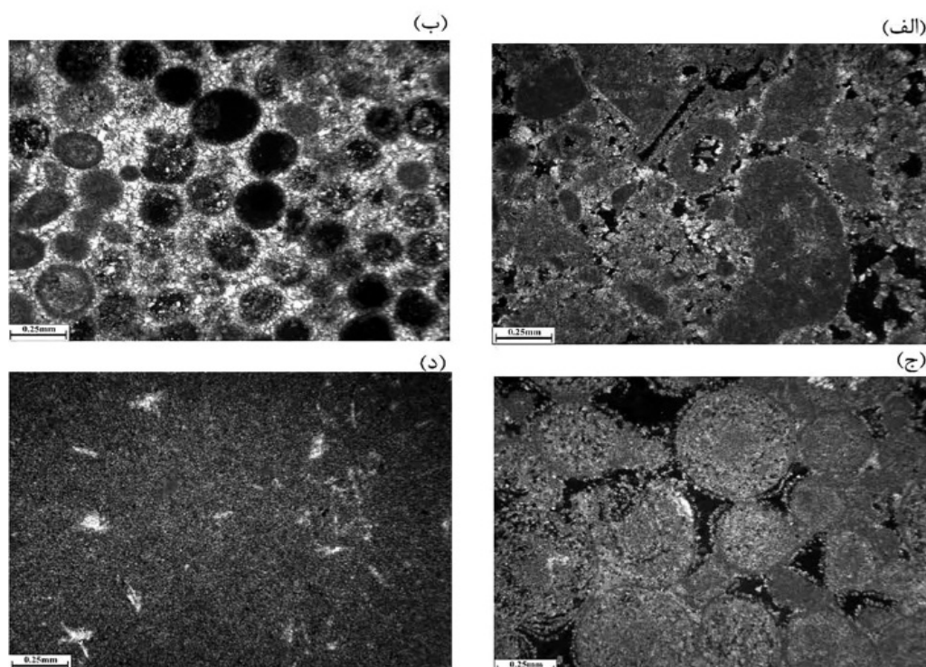
شکل ۲ تصاویری از مقطع نازک نمونه‌ها (الف) گرینستون اینتراکستی بایوکلستی دولومیتی، (ب) گرینستون با تخلخل قالبی، (ج) گرینستون با تخلخل بین دانه‌ای و (د) مادستون دولومیتی شده
