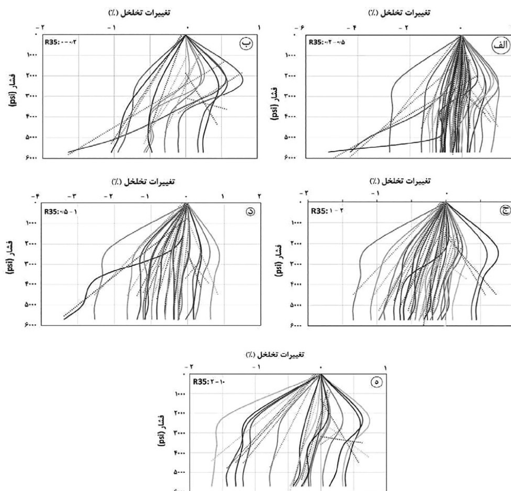
شکل ۵ نمودار تغییرات تخلخل در برابر فشار در روش وینلند در قطر گلوگاه ۰ تا ۲/الف)، ۲/ب)، ۵/ج)، ۵/د)، ۱۰ تا ۲/ه) و ۲ تا ۱۰/ه)
