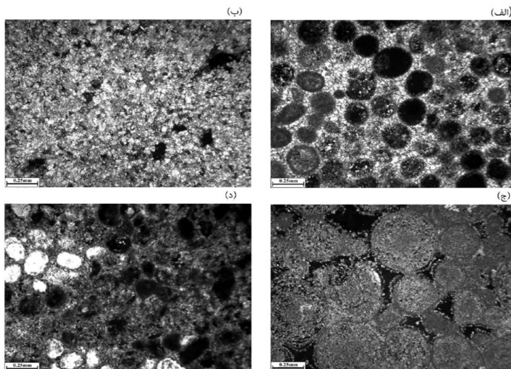
شکل ۳ نمایش فرایندهای دیاژنزی: (الف) تأثیر انحلال با گسترش تخلخل قالبی در رخساره گرینستون، (ب) دولومیتی شدن دانه‌های کربناته، (ج) سیمان دریایی اطراف دانه‌ها و (د) انحلال و تخلخل قالبی
