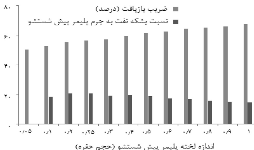
شکل ۸ ضرایب بازیافت نفت و مقدار نفت اضافه تولید شده در واحد جرم پلیمر پیش از شستشوی به کار رفته به‌عنوان تابعی از اندازه لخته پلیمر پیش از شستشو
