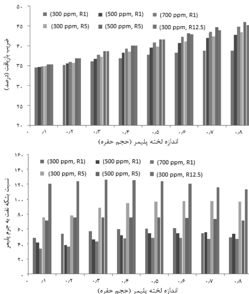
شکل ۷ نمودار (پایین) نسبت بشکه نفت اضافه تولید شده به جرم پلیمر به کار رفته به صورت تابعی از اندازه لخته پلیمر در غلظت‌ها و ضرایب مقاومت مختلف پلیمر و (بالا) ضریب باز یافت نفت برحسب اندازه لخته پلیمر برای غلظت‌ها و ضرایب مقاومت مختلف پلیمر در غلظت‌ها و ضرایب مقاومت مختلف پلیمر
