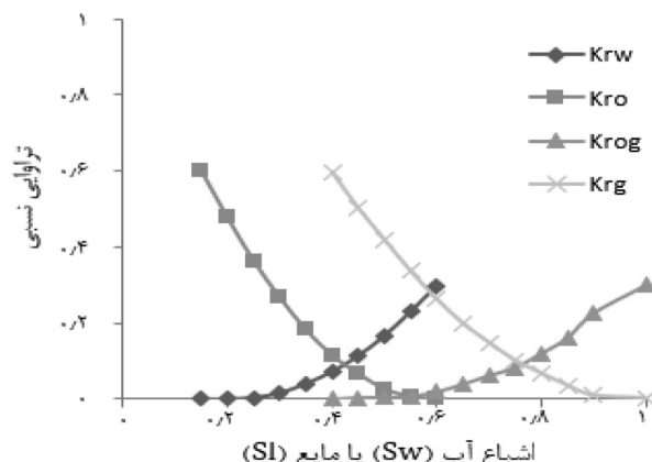
شکل ۱ نمودار تراوایی نسبی سیستم آب-نفت و مایع - گاز
