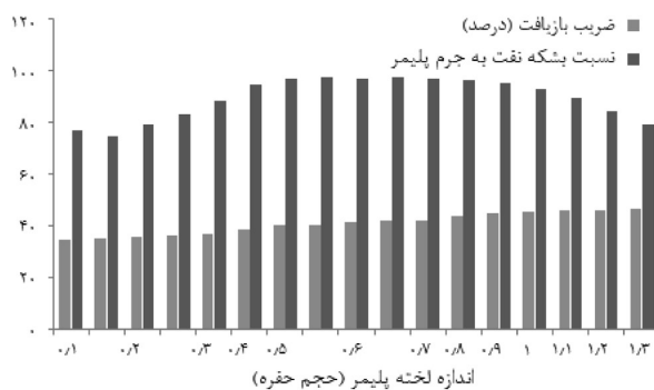
شکل ۴ ضریب بازیافت نفت و مقدار نفت اضافه تولید برحسب جرم پلیمر با اندازه لخته پلیمری با غلظت ۳۰۰ ppm و ضریب مقاومت ۵
