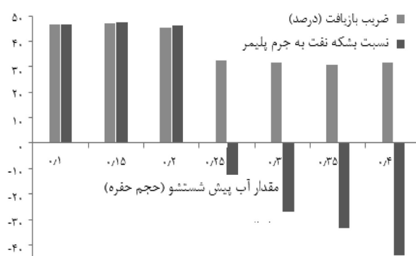
شکل ۳ ضرایب بازیافت نفت و نفت اضافه تولید شده برحسب جرم پلیمر به کار رفته از لخته‌های مختلف آب پیش از شستشو با غلظت پلیمری ppm ۵۰۰ و ضریب مقاومت ۵
