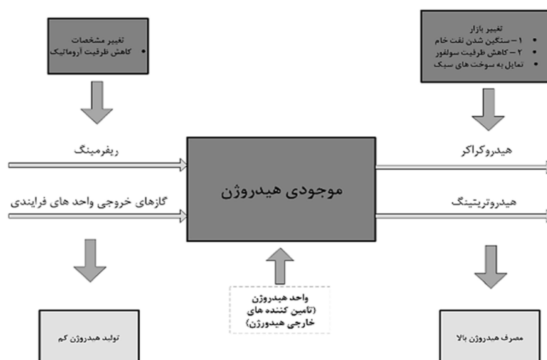
شکل ۱ نمای کلی از شبکه هیدروژن در پالایشگاه [۶]
