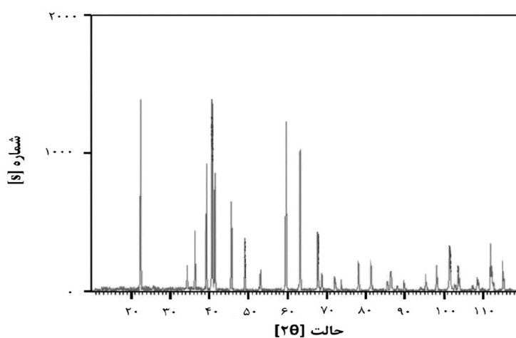
شکل ۶ نمودار XRD آلومینیوم کلرید استفاده شده در ساخت کاتالیست
