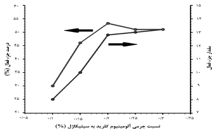
شکل ۴ اثر نسبت جرمی کاتالیست \text{AlCl}_3/\text{Silica Gel} بر مقدار جزء فعال و حذف ترکیبات گوگردی
