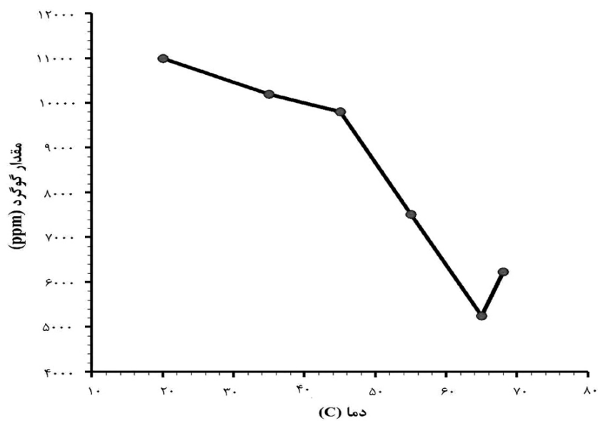
شکل ۸ بررسی اثر دماهای مختلف بر گوگردزدایی از نمونه بنزین
