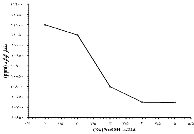
شکل ۷ بررسی اثر غلظت‌های مختلف NaOH در دمای ۶۵ °C
