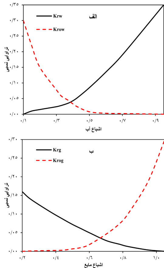
شکل ۶ نمودار تراوایی نسبی ماتریس (ترشوندگی مخلوط). الف) آب-نفت. ب) مایع-گاز.
