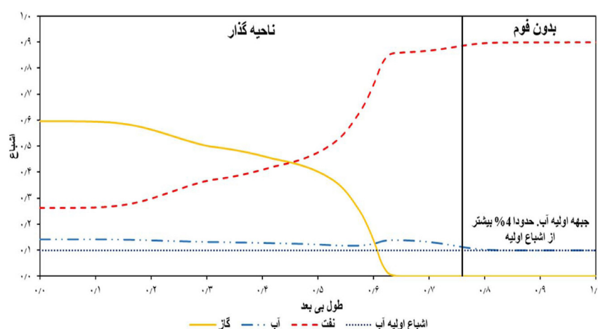
شکل ۹ پروفایل اشباع سیالات در داخل ماتریس. تراوایی نسبتاً نفت دوست و بدون فشار مؤئینه. در راستای گرید (۴,۹,۱) و پس از یک سال
