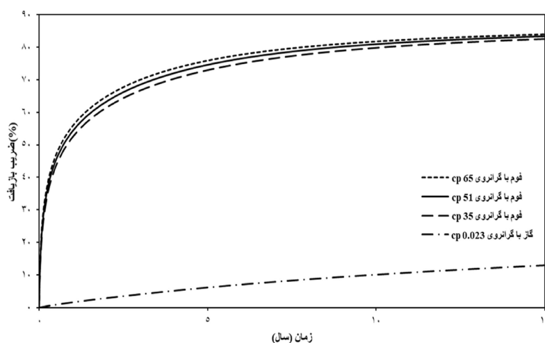
شکل ۷ تغییرات ضریب بازیافت نفت با زمان برای تزریق فوم با گرانیوی‌های مختلف در شکاف و گاز.
