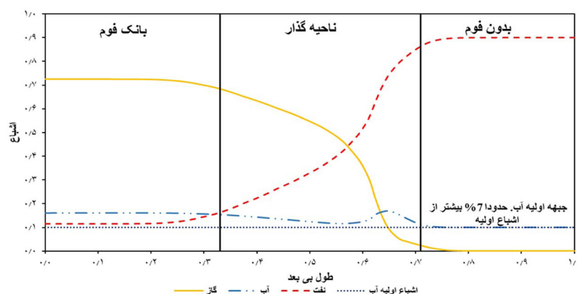
شکل ۸ پروفایل اشباع سیالات در داخل ماتریس. تراوایی نسبتاً آب دوست و بدون فشار مؤئینه. در راستای گرید (۴,۹,۱) و پس از یک سال
