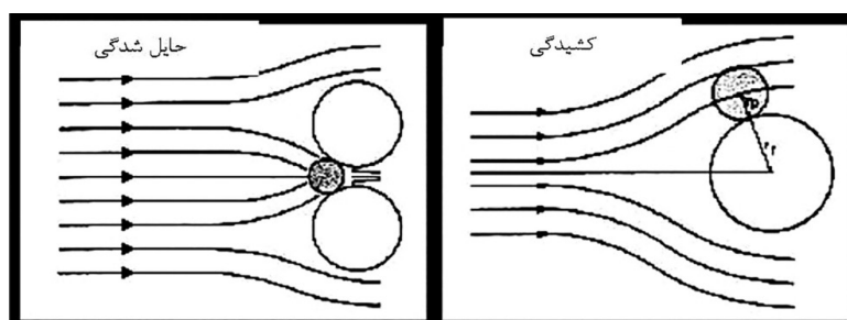
شکل ۱ شماتیک پدیده‌های کشیدگی و حایل شدگی. مکانیزم کشیدگی: قطرات بزرگی که با چسبیدن به سطح حفرات
