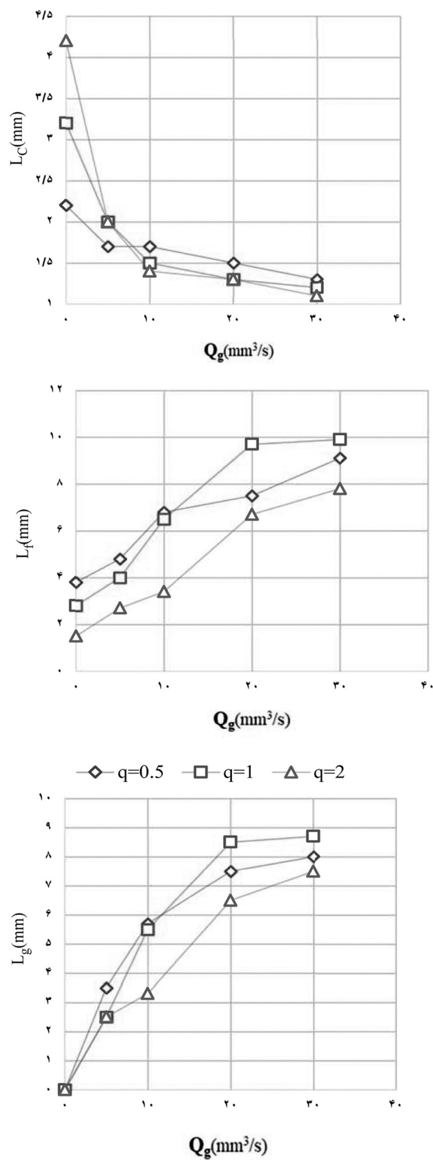
شکل ۱۰ تغییرات طول لخته‌ها نسبت به تغییرات دبی حجمی گاز برای Q_{LL}=10 \text{ mm}^3/\text{s}
