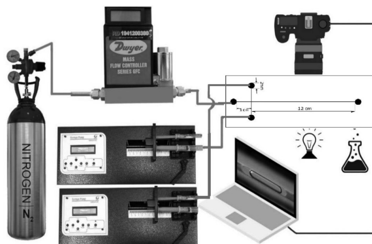
شکل ۲ شماتیک سیستم آزمایش
