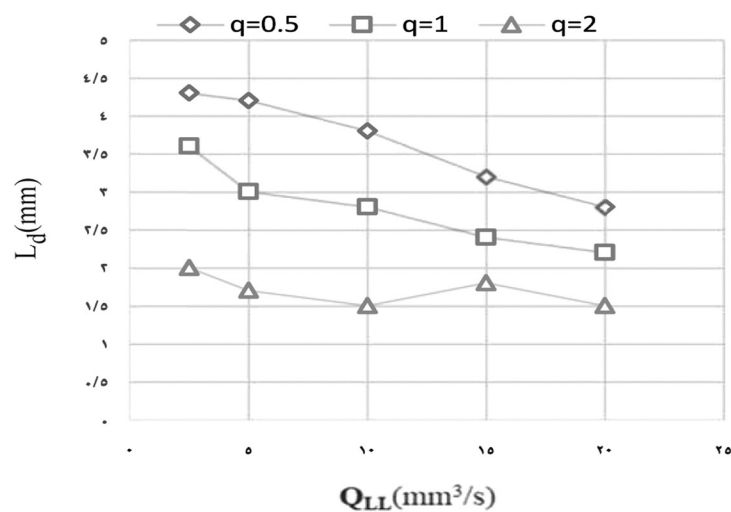
شکل ۵ تغییرات طول لخته‌های فاز آبی ( L_e ) و فاز آلی ( L_d ) با دبی جریان
