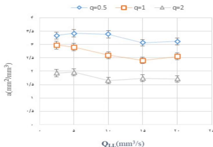
شکل ۶ تغییرات سطح بین فازي مخصوص نسبت به دبی جریان
