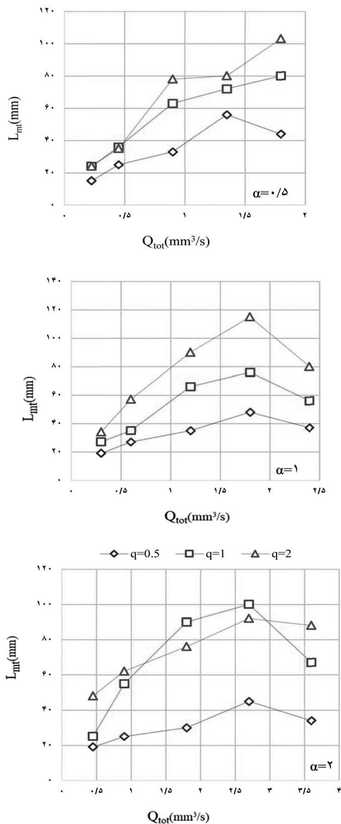
شکل ۹ وابستگی طول تغییر رنگ در حالت سه فاز به دبی فازها
