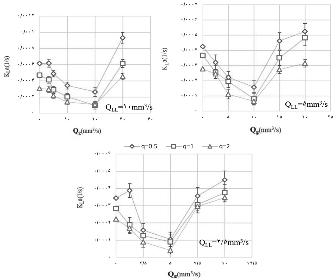
شکل ۱۳ نمودار ضریب کلی انتقال جرم برحسب تغییرات دبی جمعی گاز
