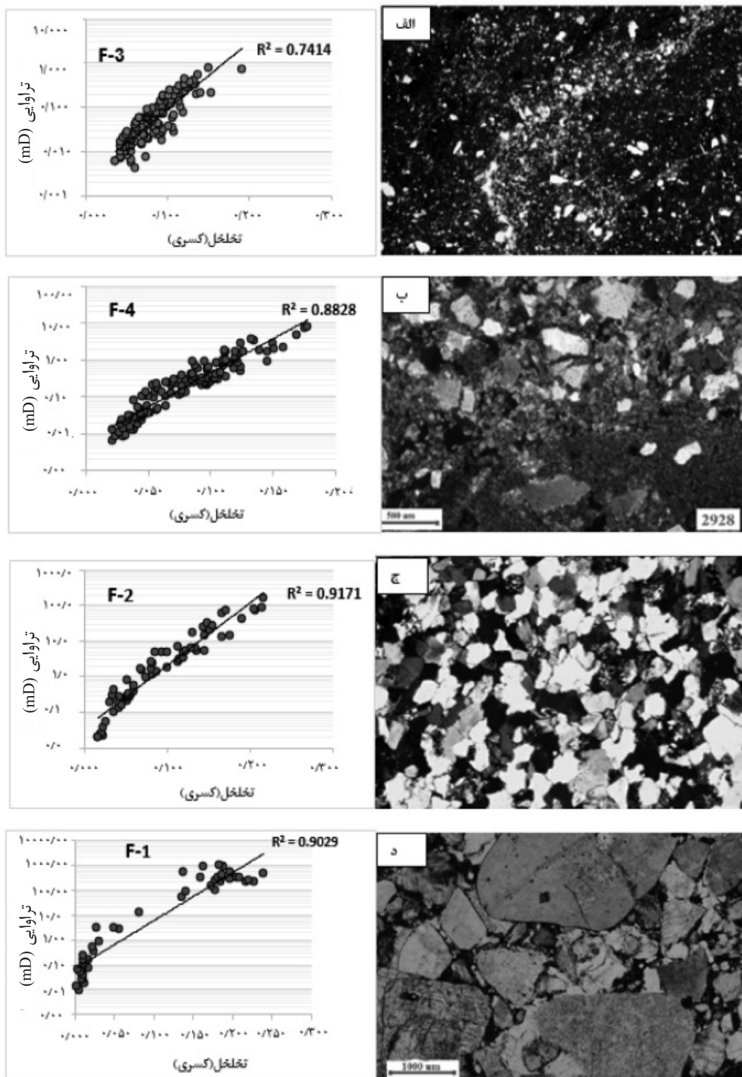
شکل ۹ نمودار تخلخل و تراوایی مغزه برای رخساره‌های شناسایی شده در سازند شورجه حوضه کپه داغ [۳]
