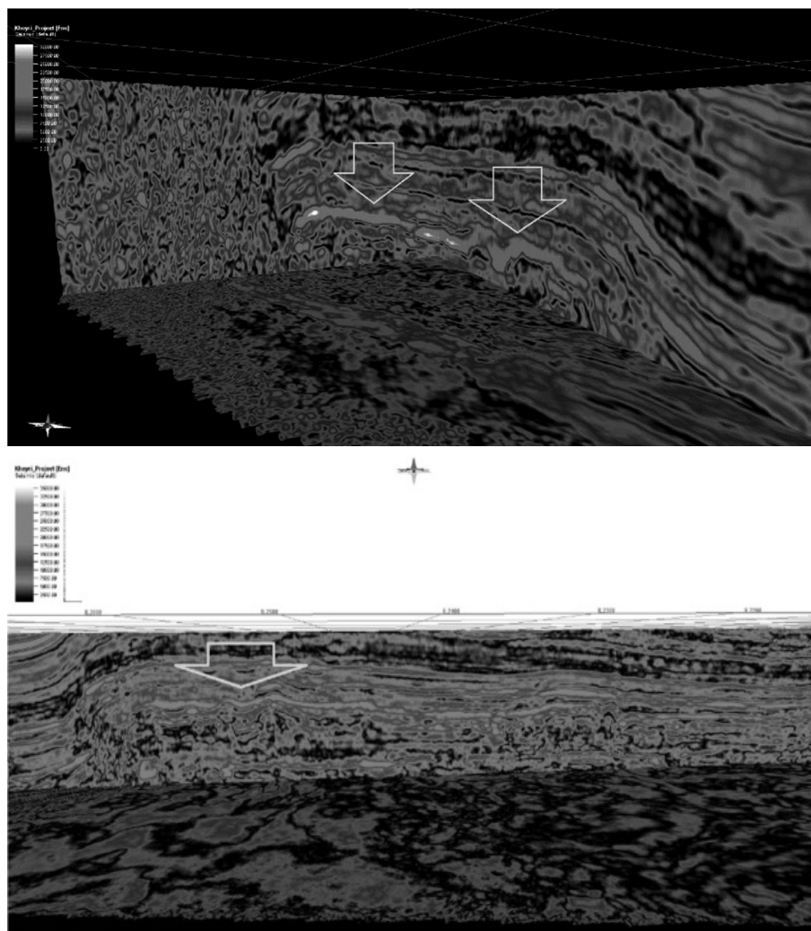
شکل ۱۵ نمایش مقاطع عرضی نشانگر پوش از مخزن شورپیجه
