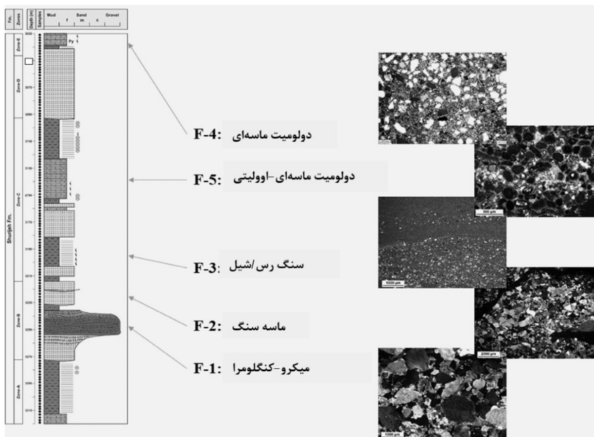
شکل ۷ توالی رسوبی و رخساره‌های مرتبط با سازند شورپیجه در میدان مورد مطالعه. پنج رخساره شامل میکروکنگلومرا، ماسه‌سنگ، رس و شیل، دولومیت ماسه‌ای و گرینستون اوئیدی در سازند شورپیجه شناسایی شده است [۳]
