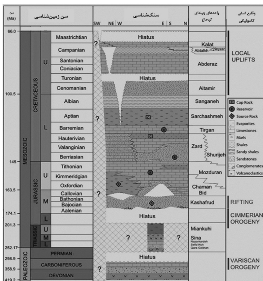
شکل ۱ ستون چینه‌شناسی حوضه رسوبی کپه داغ [۱۸]
