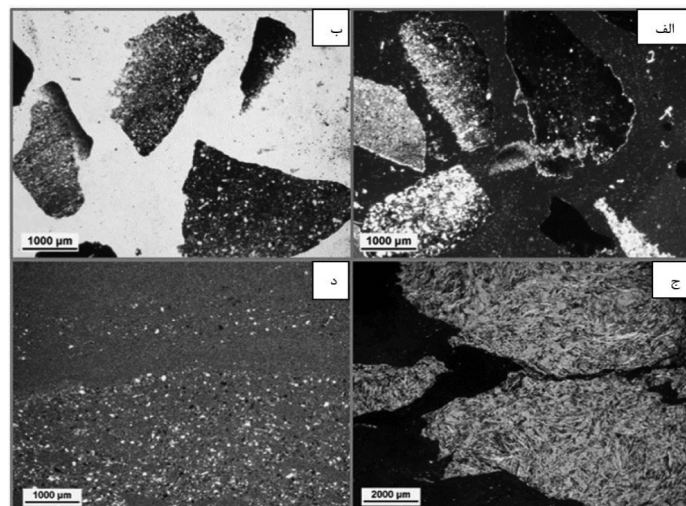
شکل ۴ تصاویر میکروسکوپی از رخساره سنگی شیل/سنگ رس به همراه رخساره مادستون با نودول انیدریت در سازند شورجه
