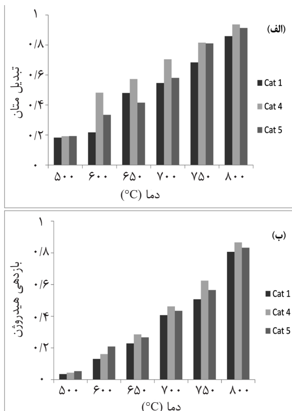
شکل ۶ ارزیابی عملکرد کاتالیست‌های سنتزی Ni / (Cat 1) و Ni-Co/Al 2 O 3 -MgO (Cat 4) با ترکیب درصد Ni/Co = ۵ و Ni-Co/Al 2 O 3 -MgO (Cat 5) با ترکیب درصد Ni/Co = ۳ و Ni/Co = ۵. الف: تبدیل متان، ب: بازدهی هیدروژن
