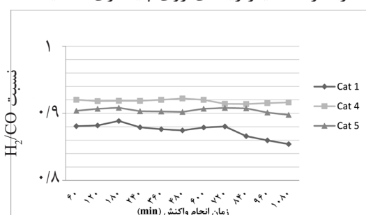
شکل ۷ تست پایداری کاتالیست‌های سنتزی Ni / Al 2 O 3 (Cat 1) و Ni-Co/Al 2 O 3 -MgO (Cat 4) با ترکیب درصد Ni/Co = ۵ و Ni-Co/Al 2 O 3 -MgO (Cat 5) با ترکیب درصد Ni/Co = ۳ و Ni/Co = ۵.
