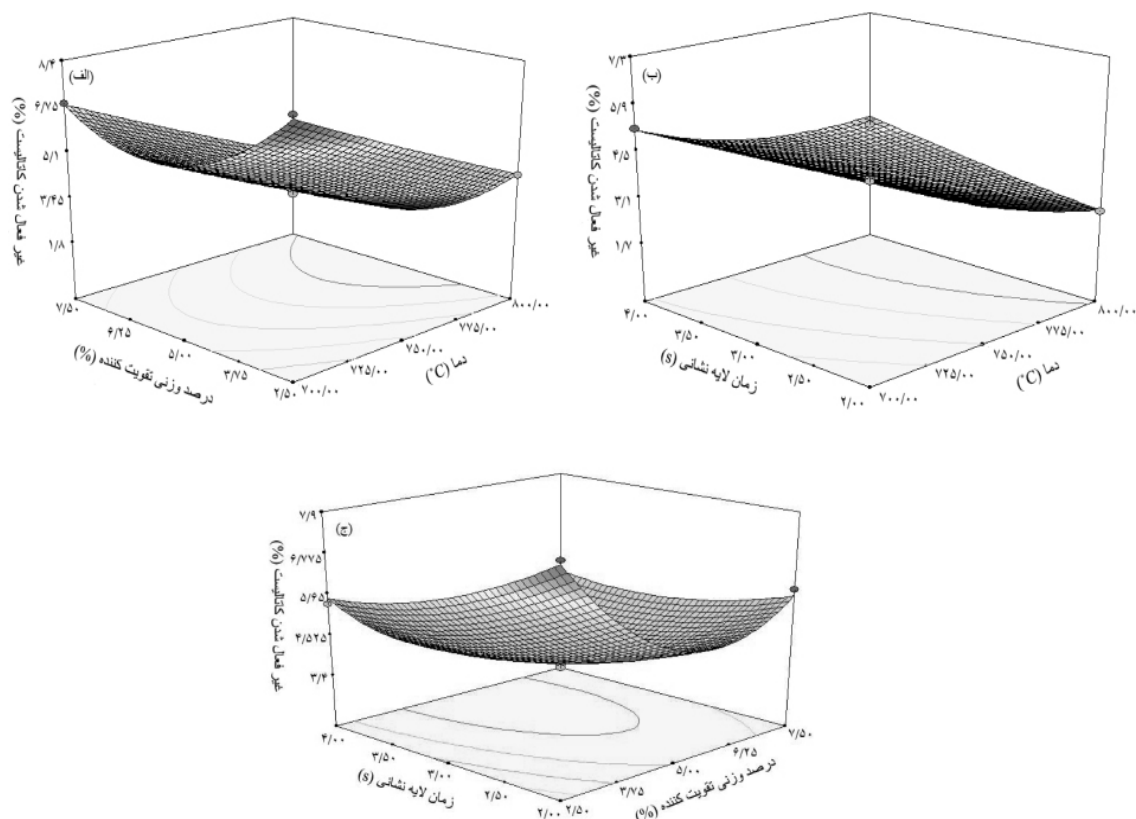
شکل ۱۰ نمودار سه بعدی و کانتور برای مدل پیش‌بینی غیر فعال شدن کاتالیست به‌عنوان تابعی از زمان لایه نشانی (t) و دمای واکنش (T) در درصد وزنی کبالت نسبت به نیکل برابر ۵٪ (ب) زمان لایه نشانی (t) و درصد وزنی کبالت نسبت به نیکل (X) در دمای واکنش ۷۵۰ °C (ج) درصد وزنی کبالت نسبت به نیکل (X) و دمای واکنش (T) در زمان لایه نشانی ۳ min
