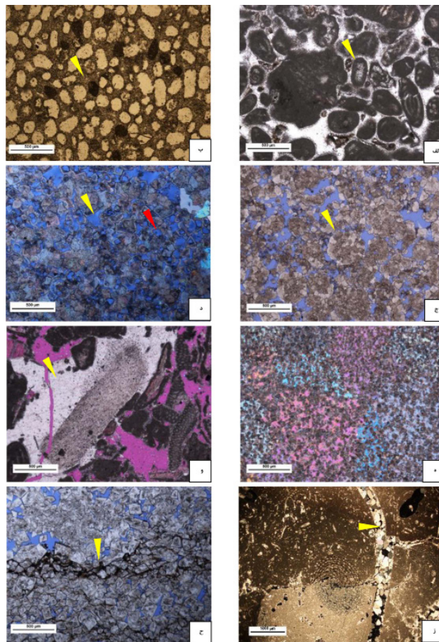
شکل ۵ تصاویر میکروسکوپی از فرآیندهای دیاژنتیکی. الف) فرآیند میکریتی شدن قطعات فسیلی. PPL. ب) دولومیتی شدن با حفظ فابریک سنگ در یک گرینستون آلییدی. انحلال باعث ایجاد تخلخل قالبی شده و سیمان انیدریتی بخشی از تخلخل‌های قالبی را پر کرده است. XPL. ج) دولومیتی شدن به صورت تخریب کننده فابریک سنگ، تنها شبحی از آلوک‌ها (آلیید) باقی مانده است. د) تخلخل بین بلوری (فلش زرد) و درون بلوری (فلش قرمز) در دولومیت‌های جان‌شینی تخریب کننده فابریک سنگ. PPL. ه) سیمان انیدریتی به صورت فراگیر بلورهای دولومیت را احاطه کرده است. و) سیمان سین تکسیال اطراف خرده اکینودرم. XPL. ز- سیمان کلسیت اسپاری بخشی از تخلخل‌های موجود را پر کرده است. PPL. ح) رگچه‌های انحلالی PPL
