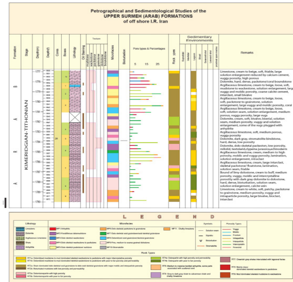
شکل ۶ ستون چینه‌شناسی، رسوب‌شناسی و پتروگرافی سازند عرب در یکی از چاه‌های میدان مورد مطالعه
