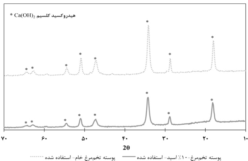
شکل ۹ الگوهای XRD پوسته تخم‌مرغ خام و پوسته تخم‌مرغ اصلاح‌شده با ۱۰٪ حجمی اسید استیک بعد از ۲۰ چرخه کربناسیون/کلسیناسیون
