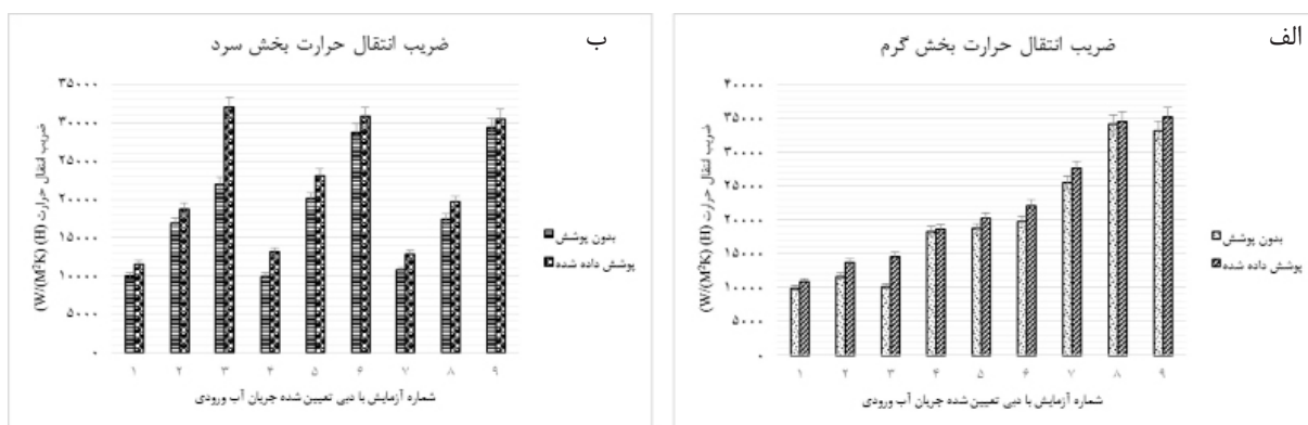
شکل ۵ مقایسه ضریب انتقال حرارت (H) برای صفحات پوشش داده شده و بدون پوشش در دو سمت الف) بخش گرم و ب) بخش سرد برای ورودی سرد 7^{\circ}\text{C} و 55^{\circ}\text{C}
