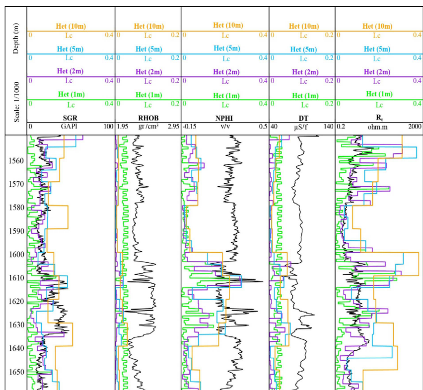
شکل ۸ فواصل ده، پنج، دو و یک متری برای نگار ناهمگنی با ضریب لورنز برای چاه A از سازند داریان.
