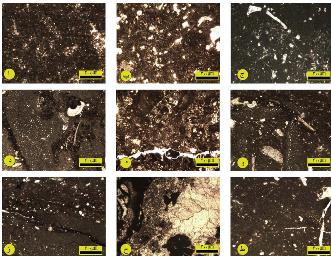
شکل ۵ تصاویر به ترتیب از چپ به راست از ا تا ط: دولومیتی شدن، میکرایتی شدن، زیست‌آشفته‌گی، انحلال، نوشکلی، تراکم فیزیکی، استیلولیت، سیمان (بلوکی) و شکستگی. همه تصاویر در نور طبیعی تهیه شده است.
