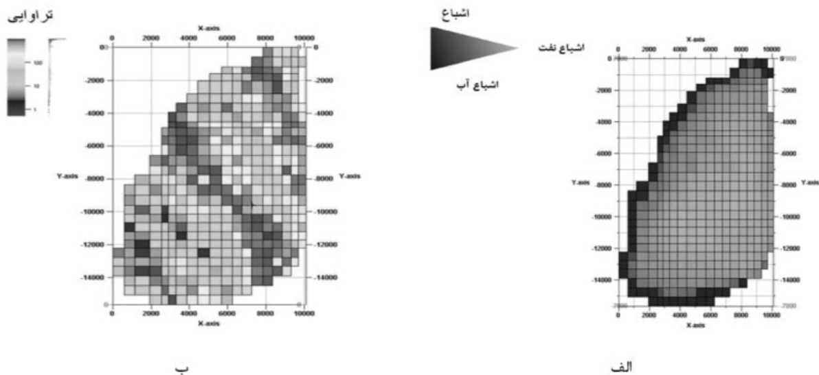
شکل ۷ الف) توزیع اشباع آب (ب) توزیع تراوایی در مدل PUNQ-S3.
