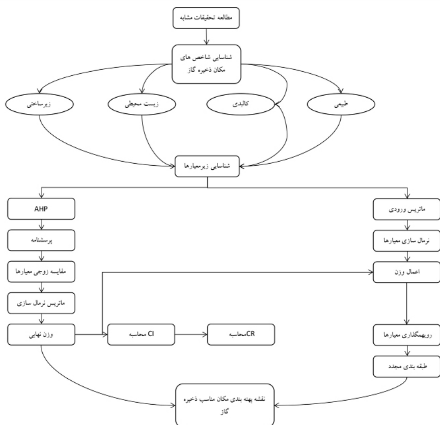
شکل ۳ فرآیند مکان‌یابی ذخیره گاه گازی
