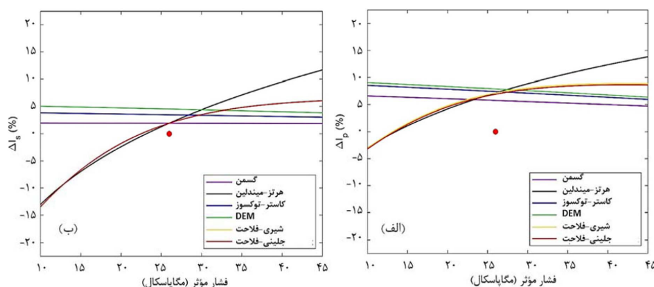
شکل ۱ (الف) تغییرات مقاومت صوتی موج تراکمی و (ب) تغییرات موج برشی در اثر جانشینی ۷۰٪ از نفت مخزن با آب به ازای مقادیر مختلف فشار موثر.
