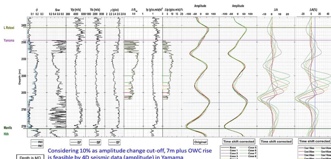
شکل ۶ نگاره‌های دامنه و تغییرات آن برای حالت‌های مختلف بالا آمدگی سطح تماس آب و نفت در چاهی در مخزن یاماما.
