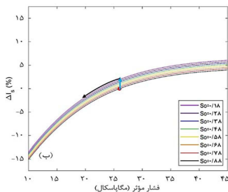
شکل ۳ نمایش تغییرات (الف) مقاومت صوتی تراکمی ( \Delta I_p ) و (ب) مقاومت صوتی برشی ( \Delta I_s ) در اطراف چاه تولیدی و تزریقی در مقابل تغییر فشار مؤثر برای جانشینی ۷۰٪ از نفت توسط آب طی فرآیند تزریق آب سازندی به مخزن.
