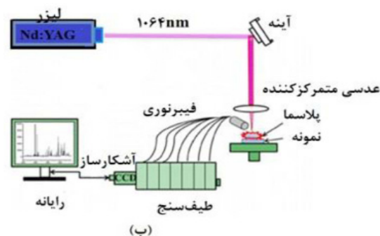
شکل ۱ الف) دستگاه تجاری، ب) چیدمان آزمایشگاهی دستگاه LIBS
