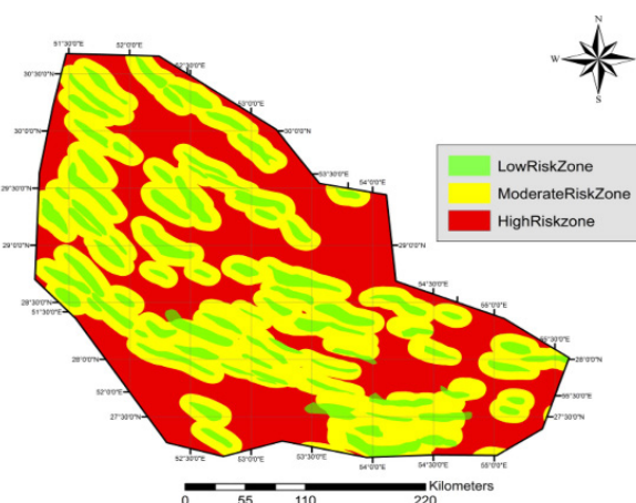
شکل ۸ نقشه نهایی ریسک زمین‌شناسی
