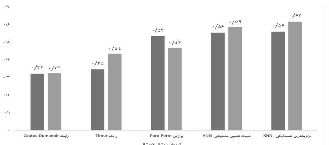
شکل ۸ مقایسه ضریب همبستگی روش‌های مورد استفاده در تخمین تراوایی به تفکیک لایه‌های ۱ و ۲ و لایه ۳ در چاه C
