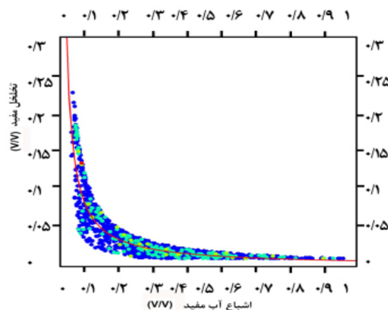
شکل ۲ نمودار تقاطعی تخلخل به اشباع آب در بخش‌های مخزنی چاه‌های حاوی اطلاعات مغزه
