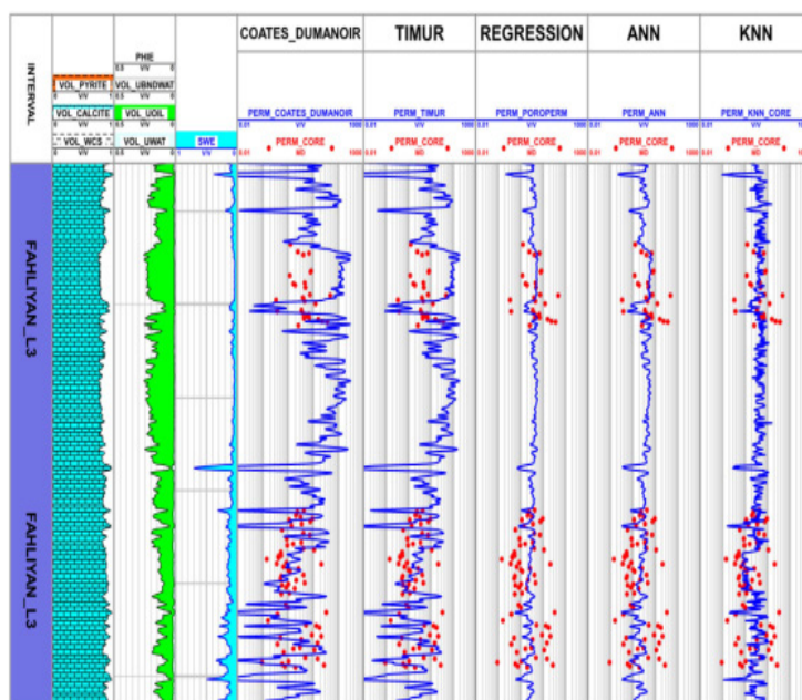
شکل ۷ مقایسه تراوایی حاصل از روش‌های مختلف و نقاط تراوایی مغزه، لایه ۳ فهلین، چاه C
