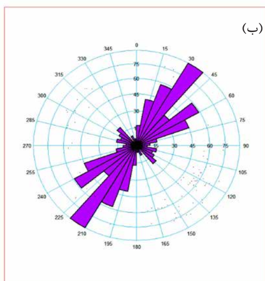
شکل ۱۴ جهت شکستگی‌ها در مخزن بخش بالایی (با تعداد بیشتری از شکستگیها) (الف) و بخش پایینی (با تعداد کمتری از شکستگی‌ها) (ب)
