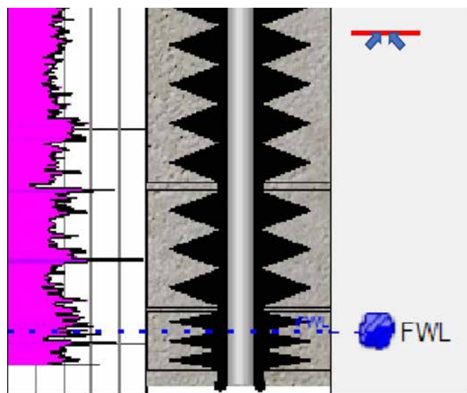
شکل ۱ نشتی لوله‌های پوششی و راه‌یابی آب به چاه تولیدی
