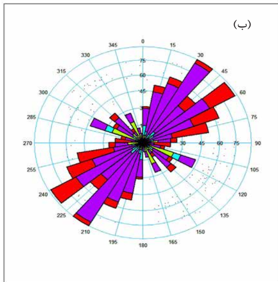
شکل ۱۳ شیب (الف) و جهت (ب) شکستگی‌ها در ناحیه مورد مطالعه
