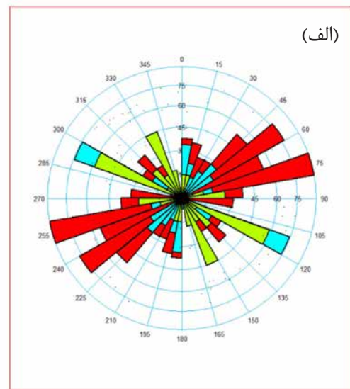
شکل ۱۴ جهت شکستگی‌ها در مخزن بخش بالایی (با تعداد بیشتری از شکستگیها) (الف) و بخش پایینی (با تعداد کمتری از شکستگی‌ها) (ب)
