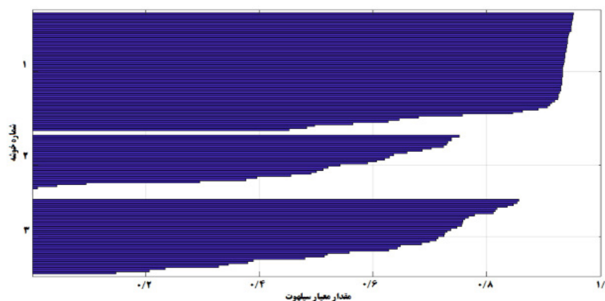
شکل ۴ معیار سیلپوت برای نواحی کاندیدا
