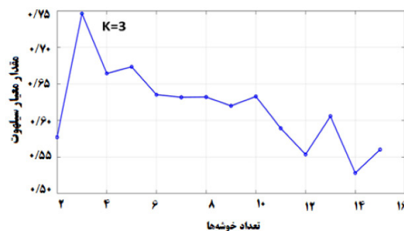
شکل ۵ تعیین تعداد خوشه بهینه با توجه به معیار سلیهوت
