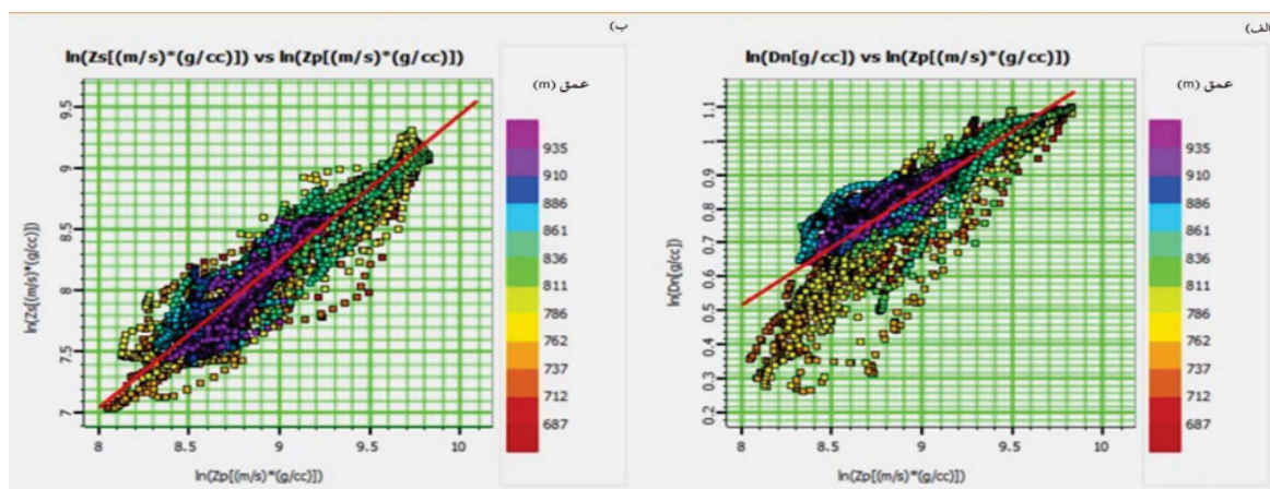
شکل ۷ رابطه خطی بین مقاومت تراکمی و چگالی-مقاومت تراکمی. الف) نشان دهنده برازش خطی در ترسیم متقاطع \ln(D_n) و \ln(Z_p) می باشد. ب) رابطه بین مقاومت برشی و مقاومت تراکمی که از برازش خطی در ترسیم متقاطع \ln(Z_s) و \ln(Z_p) به دست می آید
