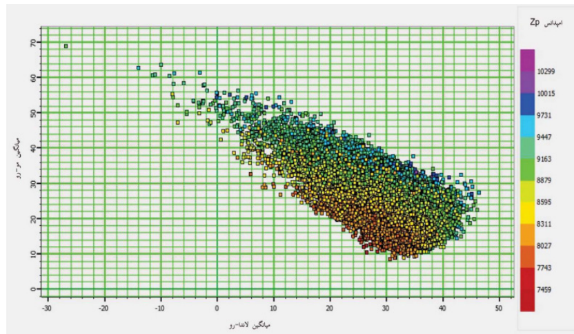
شکل ۱۶ نمودار مقاطع \lambda\rho - \mu\rho نشان‌دهنده توزیع یکسان اشباع یک نوع سیال
