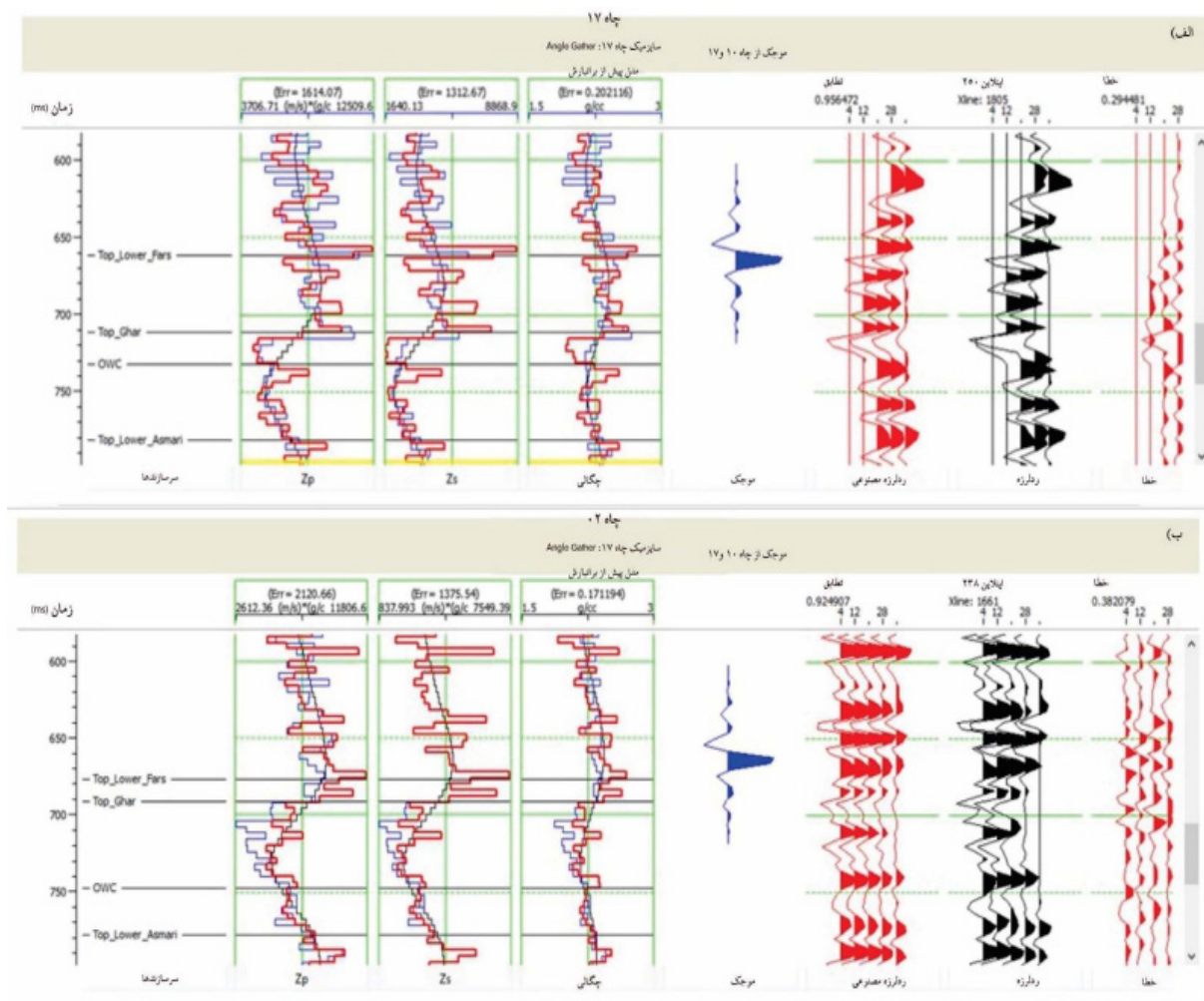
شکل ۸ نتیجه وارون‌سازی در محل چاه الف (شماره ۱۷ و ب) شماره ۲
