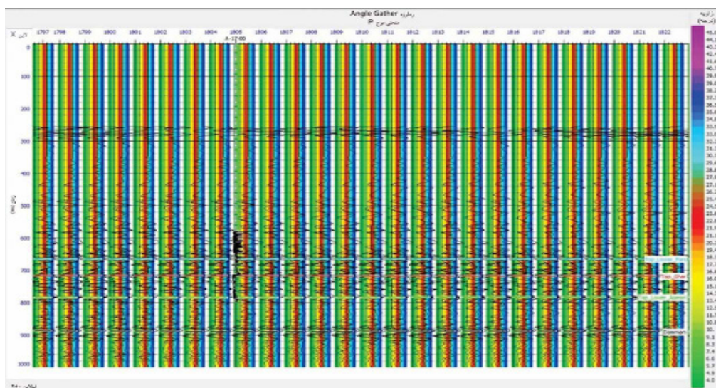
شکل ۴ نمایش Angle Gather به دست آمده جهت انجام مطالعات AVO با طیف رنگی زاویه تابش در اطراف چاه A-۱۷
