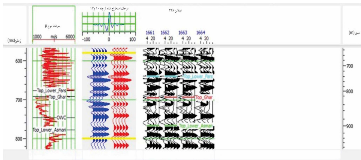
شکل ۲ تطابق چاه A-۰۲ با استفاده از موجک استخراج شده از اطلاعات چاه و لرزه (ضریب همبستگی ۷۲٪)
