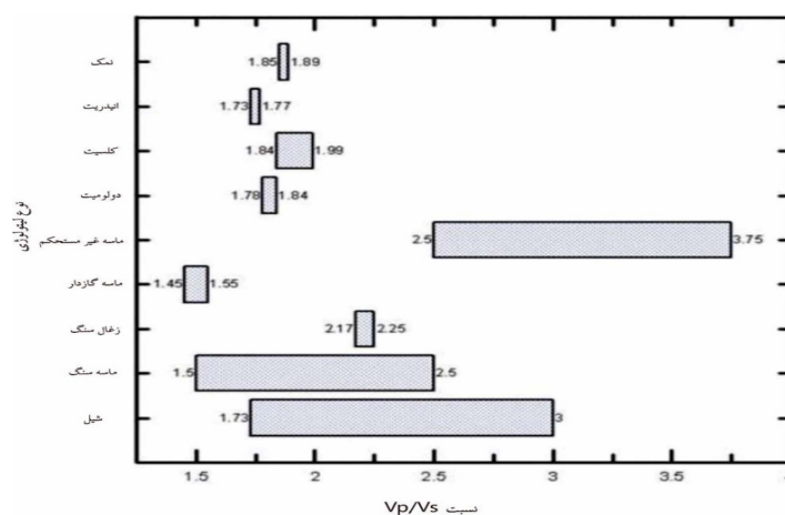
شکل ۱۷ تعیین لیتولوژی با استفاده از روش نسبت سرعت‌ها [۳۲]
