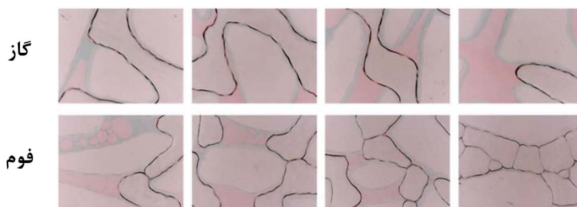
شکل ۸ تصاویر میکرومقیاس در خصوص نحوه توزیع و اندازه حباب‌های گاز در طول تزریق گاز و تزریق فوم در حفرات محیط متخلخل
