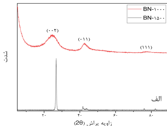
شکل ۲ مقایسه الف) الگوی پراش پرتو ایکس [۲۵] و ب) طیفسنجی رامان از نمونه نیتريدبور سنتز شده در دماهای ۱۰۰۰ °C و ۱۵۰۰ °C
