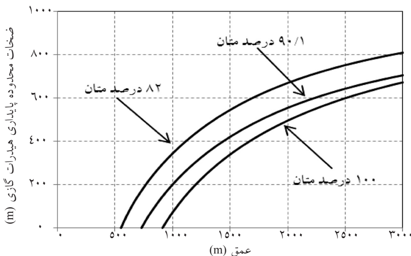
شکل ۶- ضخامت محدوده پایداری هیدرات گازی بر حسب عمق آب برای سه ترکیب گازی
