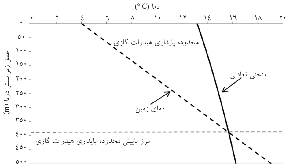
شکل ۲- محدوده پایداری هیدرات در رسوبات دریایی (دمای بستر 4^{\circ}\text{C} ، گرادیان 20^{\circ}\text{C}/\text{km} ، فشار هیدروستاتیک خطی 10\text{ MPa}/\text{km} و عمق آب 1000\text{ m} ) [۲۸]. (محل تقاطع منحنی تعادلی و دمای زمین مرز پایینی محدوده پایداری بوده و ضخامت آن را نمایش می‌دهد)
