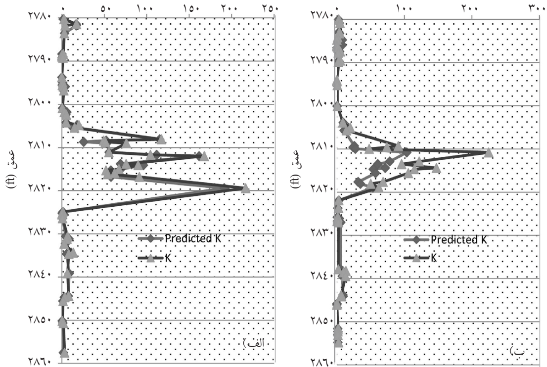
شکل ۷- نمودار مقایسه تراوایی مغزه و تراوایی پیش‌بینی شده برحسب عمق داده‌های آموزشی در چاه شماره ۳ با روش ACE برای داده‌های آموزش و (ب) داده‌های تست (الف)
