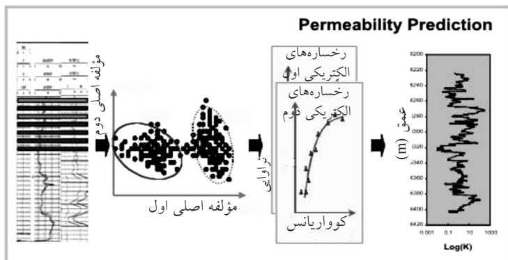
شکل ۳- نمودار طرح‌واره از پیش‌بینی تراوایی با شناسایی الکتروفاسیس‌ها
