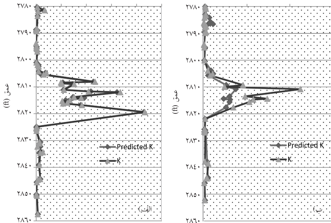
شکل ۸- نمودار مقایسه تراوایی مغزه و تراوایی پیش‌بینی شده برحسب عمق داده‌های آموزشی در چاه شماره ۳ با روش شبکه عصبی برای داده‌های آموزش و (ب) داده‌های تست (الف)
