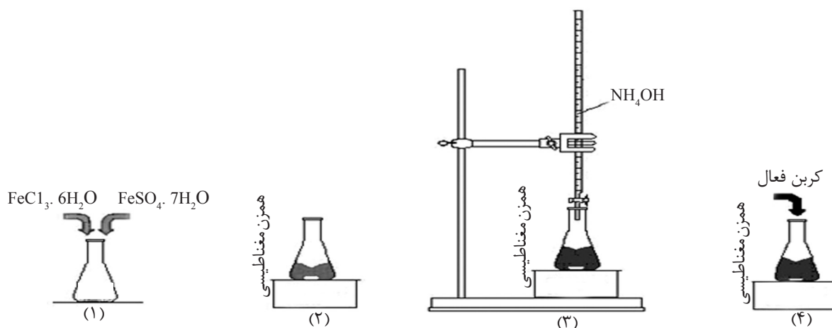
شکل ۱- نمای شماتیک از مغناطیس کردن کربن فعال به روش اضافه کردن کربن فعال حین تولید نانوذرات (۱) افزودن مواد اولیه، (۲) حل کردن نمک های آهن، (۳) جوانه زنی فاز مگنتیت و (۴) افزودن کربن فعال
