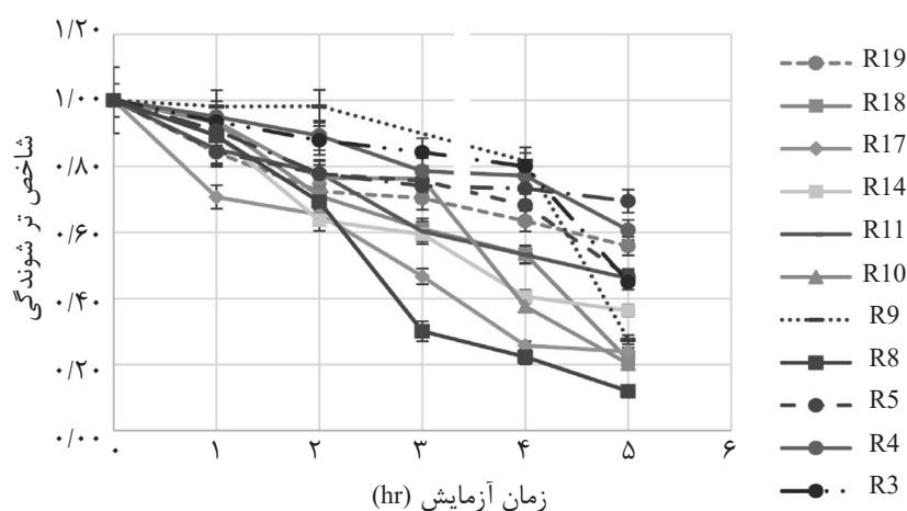
شکل ۷ نمودار ترشوندگی در برابر زمان برای نمونه‌های مختلف نانوسیال
