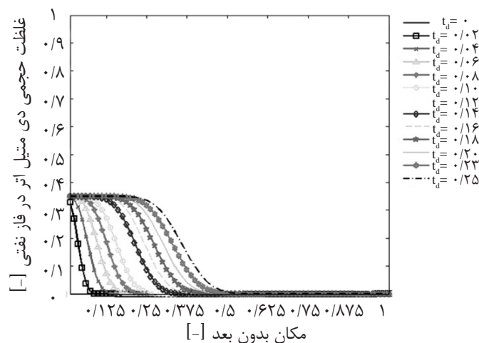
شکل ۳ پروفایل غلظت دی متیل اثر در فاز نفتی براساس مکان بدون بعد در طول فرآیند DEW تا زمان t_d = 0.25
