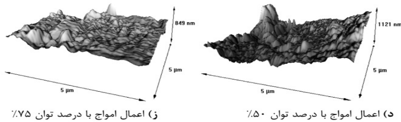
شکل ۱۳ تصاویر AFM از تاثیر امواج فراصوت بر کاهش رسوبات نانوذرات
