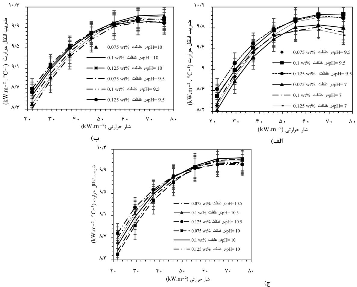
شکل ۸ تاثیر pH بر ضریب انتقال حرارت در جوشش نانوسیال: الف) ۹/۵، ب) ۹/۵ و ۱۰ (ج) ۱۰ و ۱۰/۵
