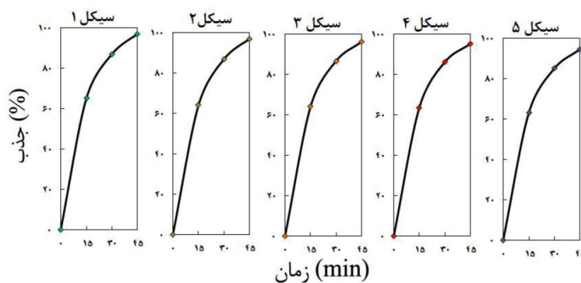
شکل ۱۰ کارایی جذب DBT در حضور جاذب TMU-11NP پس از پنج چرخه در مدت ۴۵
