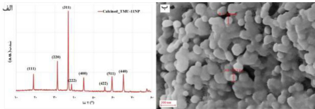
شکل ۱۱ الگوی PXR (الف) و تصویر SEM (ب) از ساختار مکعبی \text{Co}_3\text{O}_4 تهیه شده به روش کلسینه کردن TMU-11NP در دمای 600^\circ\text{C}
