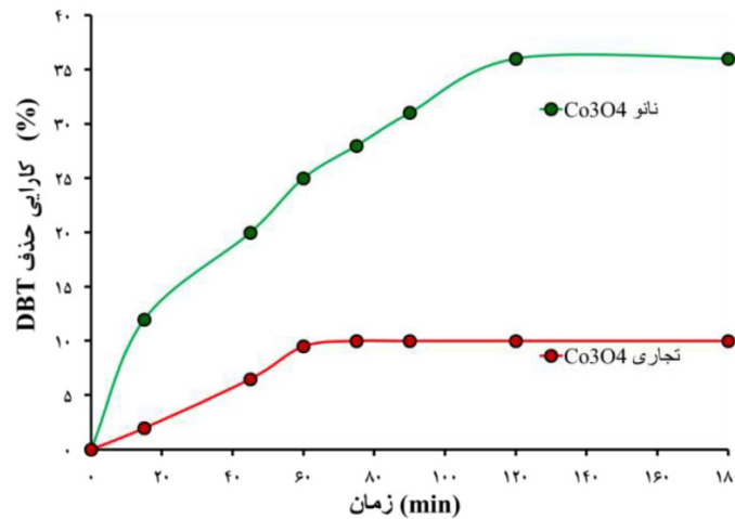
شکل ۱۲ راندمان حذف DBT در حضور ۳۰ mg نانوساختار \text{Co}_3\text{O}_4 و \text{Co}_3\text{O}_4 تجاری در دمای 60^\circ\text{C}
