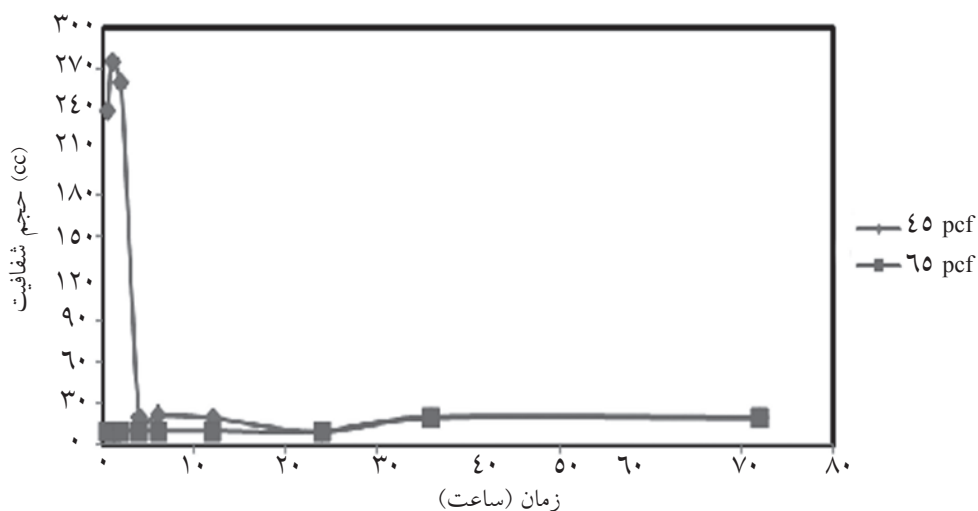
شکل ۳- مقایسه حجم رسوبات شفاف سیالات حفاری با دانسیته 45 و 65 \text{ lb/ft}^3 رقیق شده با آب دریا به نسبت 2:3
