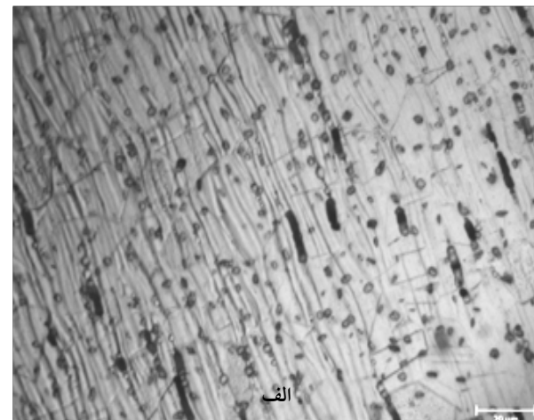
شکل ۲- ساختار میکروسکوپی آلیاژ ۳۱۶L عملیات حرارتی شده در ۸۰۰ °C به مدت ۳ ساعت، الکترواچانت: اسید اگزالیک ۱۰ درصد الف: مقطع طولی ب: مقطع عرضی
