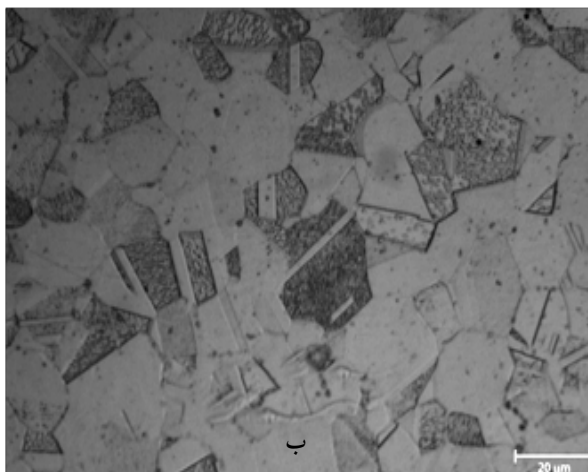
شکل ۲- ساختار میکروسکوپی آلیاژ ۳۱۶L عملیات حرارتی شده در ۸۰۰ °C به مدت ۳ ساعت، الکترواچانت: اسید اگزالیک ۱۰ درصد الف: مقطع طولی ب: مقطع عرضی
