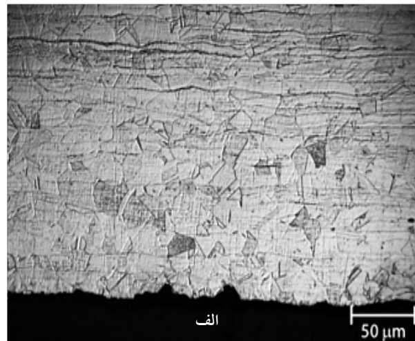
شکل ۱- ساختار میکروسکوپی سطح نمونه‌های عملیات سطحی شده، الکترواچانت: اسید اگزالیک ۱۰ درصد الف: سند بلاست شده ب: شات بلاست شده
