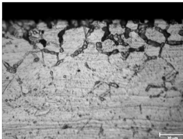
شکل ۳- ساختار میکروسکوپی عمق حساس شدگی آلیاژ ۳۱۶L عملیات حرارتی شده در ۸۰۰ °C به مدت ۳ ساعت، الکترو اچانت: اسید اگزالیک ۱۰ درصد
