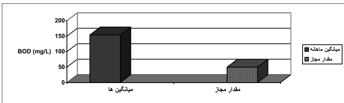
شکل ۱۴- مقایسه میزان اکسیژن خواهی زیستی پساب خروجی واحد پارازیلن با مقادیر مجاز
