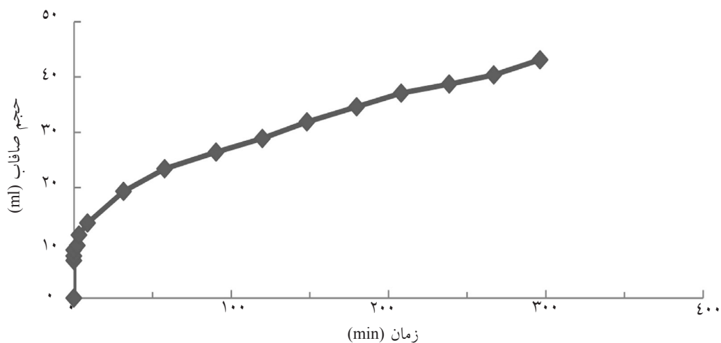
شکل ۶ الف- صافاب دینامیکی بر حسب زمان (۰/۵٪ ذرات الیافی در گل و عرض شکاف 221 \mu\text{m} ).
