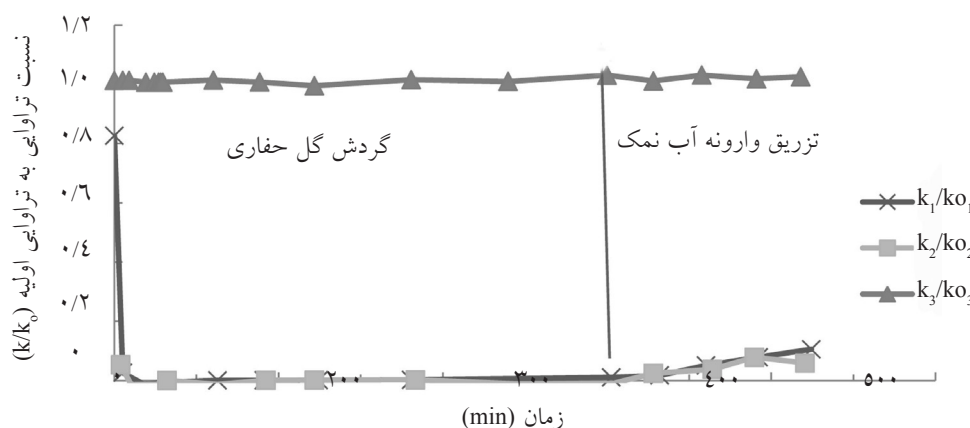
شکل ۱۴- میزان آسیب تراوایی شکاف بر حسب زمان (عرض شکاف 207 \mu\text{m} )
