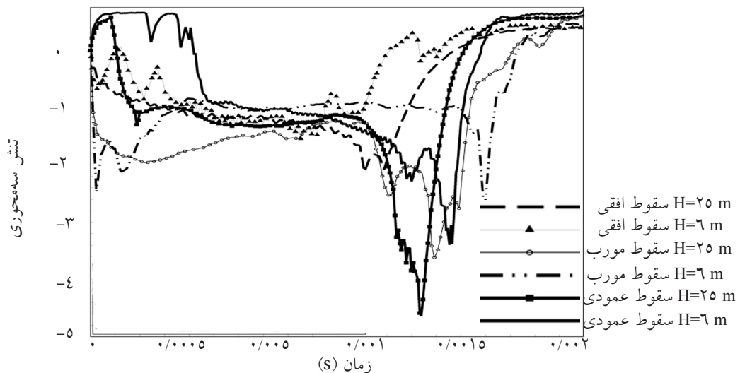
شکل ۲۱- تغییرات زمانی تنش سهمحوری در نقطه‌ای از ناحیه آسیب دیده برای سقوط در فشارکاری
