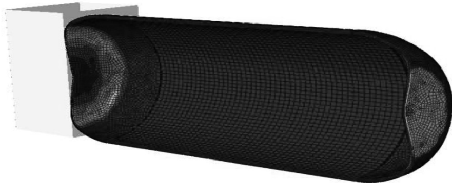
شکل ۲- مدل تغییر شکل یافته مخزن پس از تصادم عمودی
