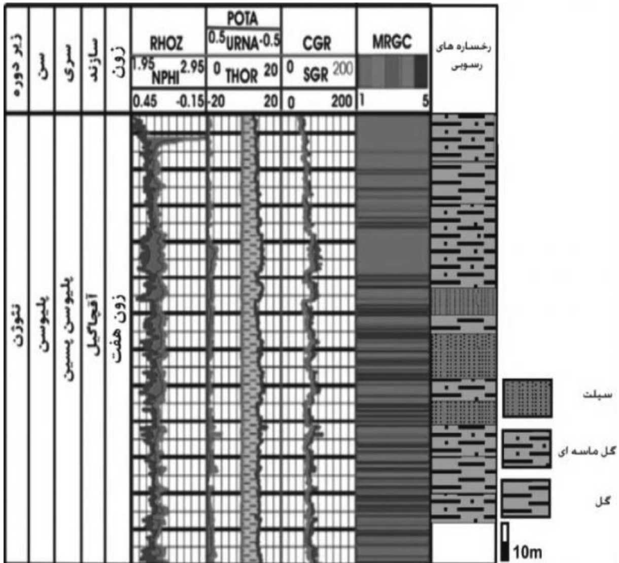
شکل ۱۳ لاگ‌های پتروفیزیکی و الکتروفاسیس‌های زون ۷ سازند آقچاگیل.
