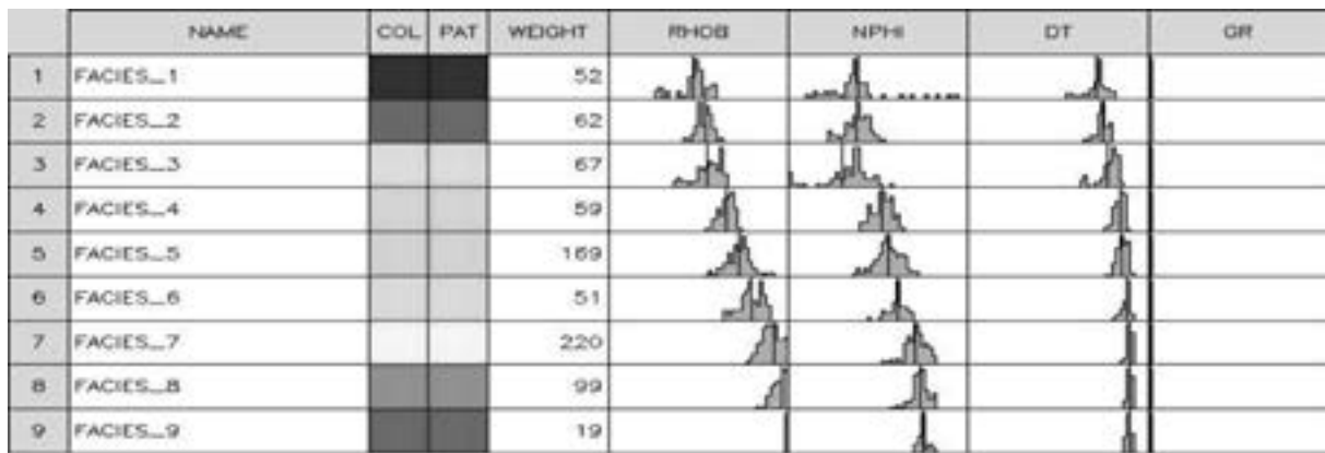
شکل ۴ خوشه‌سازی با روش MRGC.
