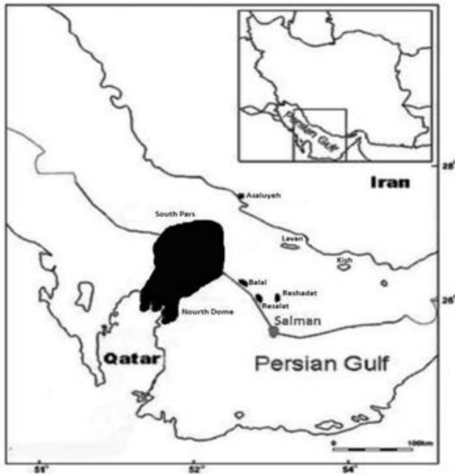
شکل ۱ موقعیت جغرافیایی میدان نفتی سلمان [۲].
